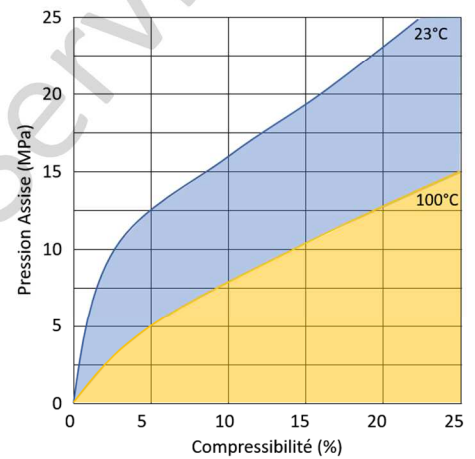
Courbe de compression sous contrainte en température
